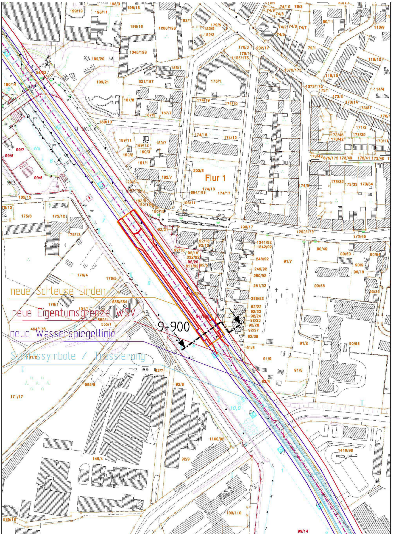
LAGEPLAN zur Lage der neuen Schleuse für den Stichkanal Linden im oberen Vorhafen, südöstlich vorhandener Schleuse - einschließlich Flächenansprüche der WSD Mitte im Bereich der Dieselstraße / Planungsstand Jan. 2009
