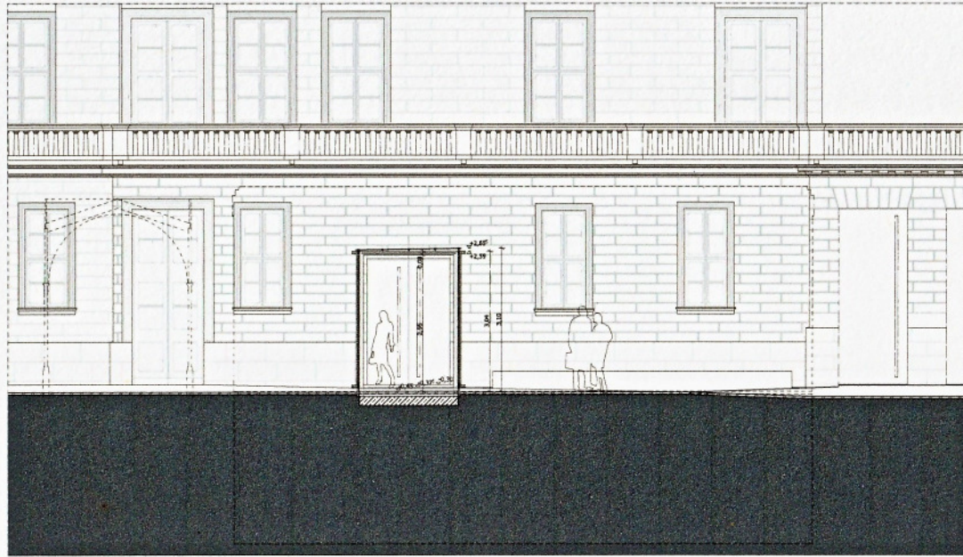
Querschnitt
