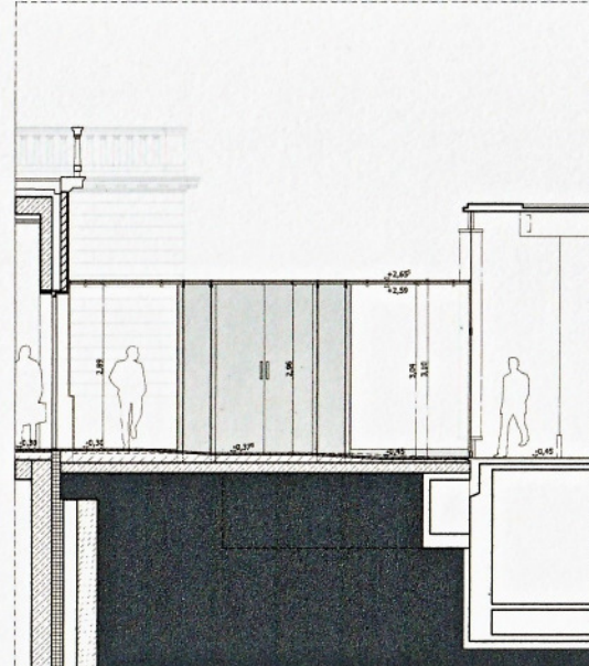
Längsschnitt
