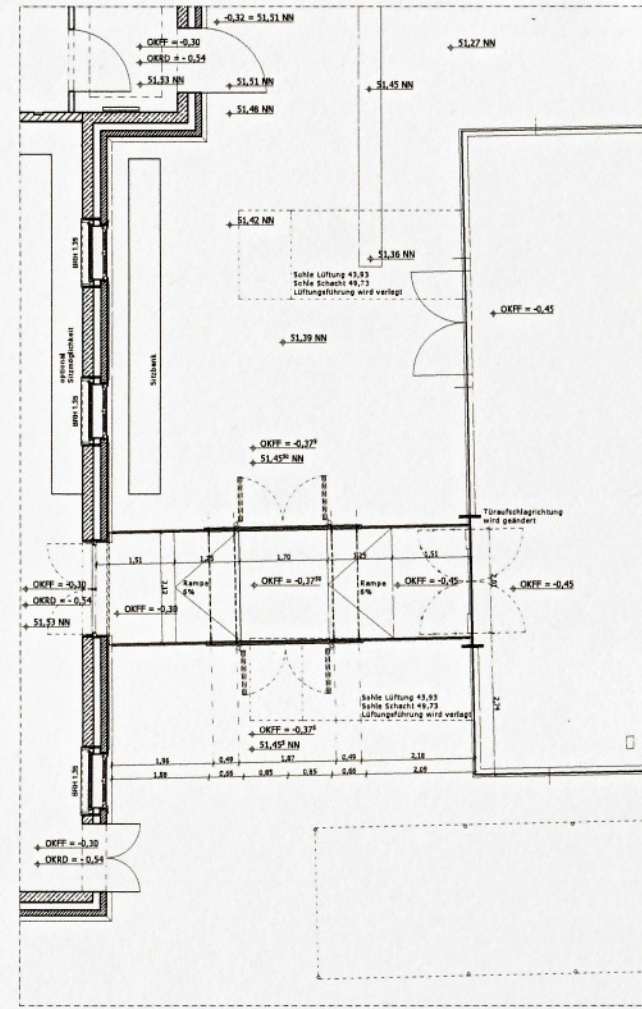
Grundriss
