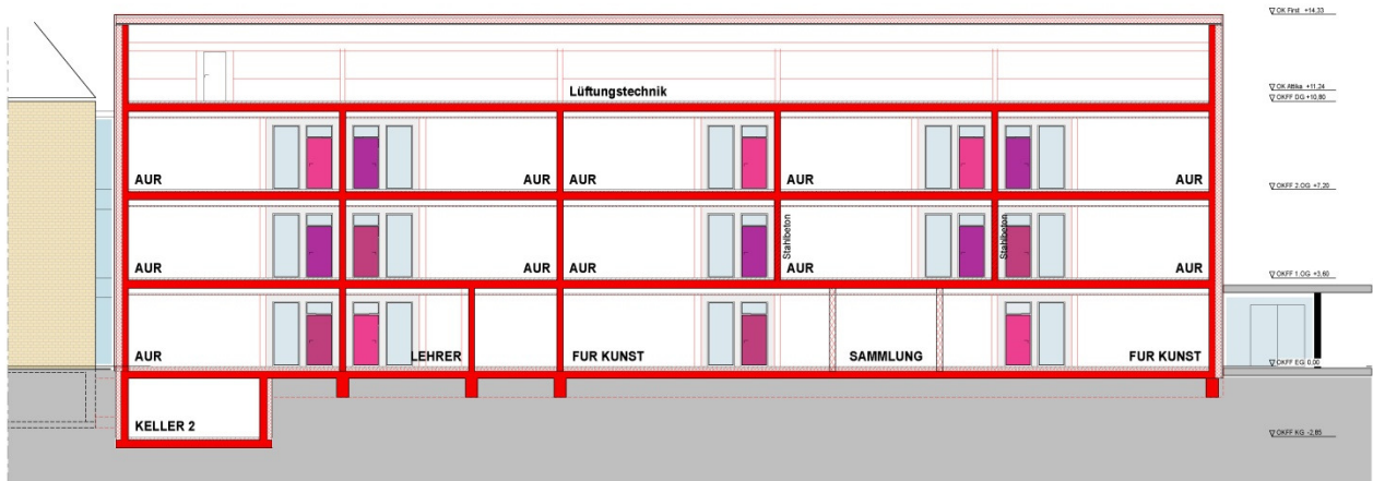
SCHNITT c_c
