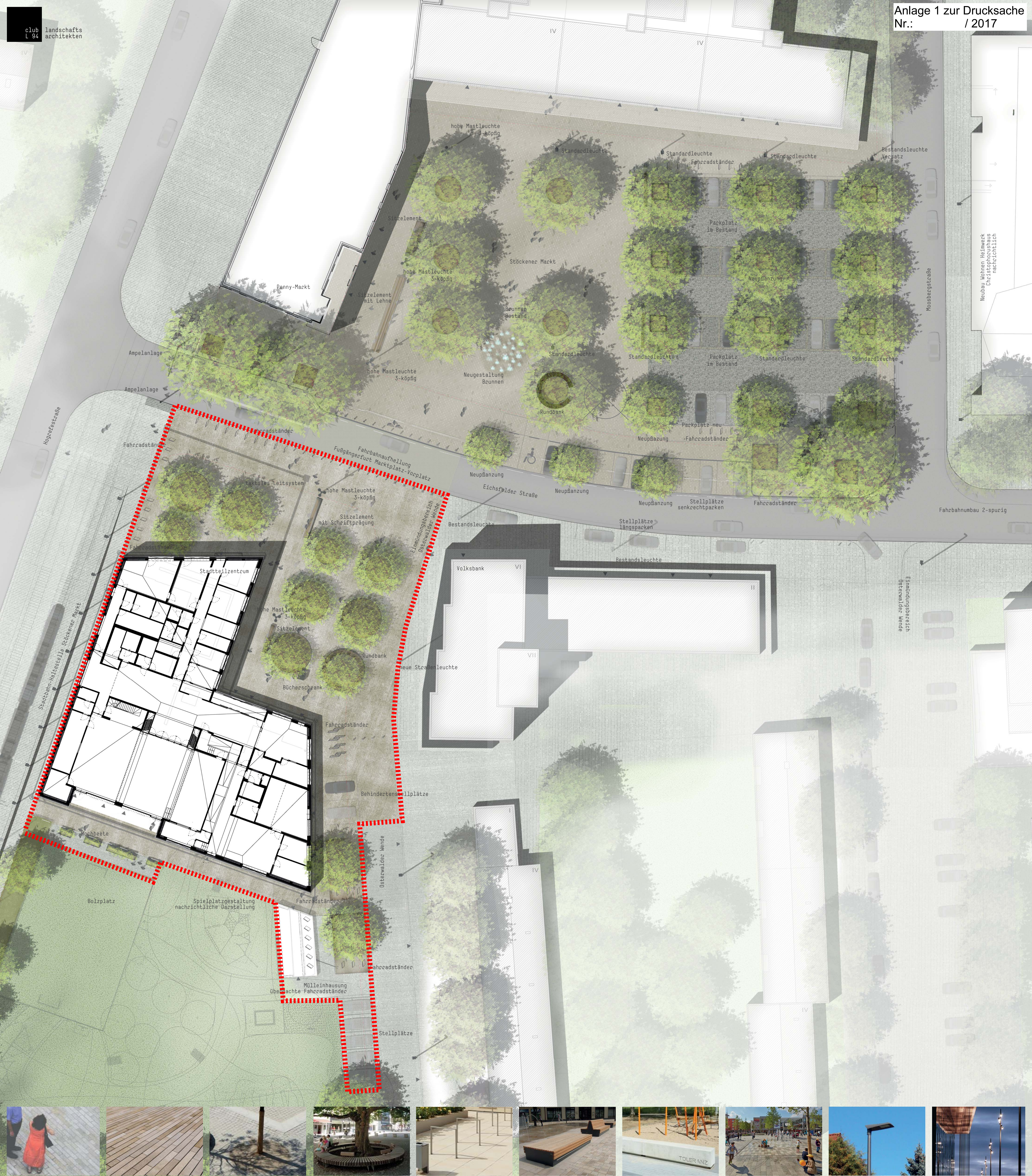
Betonplattenbelag Stadtmarkt, Wassergeb. Wegedecke - Baumscheiben - Rundbank, Fahrradlehnenbügel, Sitzelement mit Holzauflage, Sitzelement mit Schriftprägung, Neugestaltung Brunnen, Standardleuchte LHH, Mastleuchte
