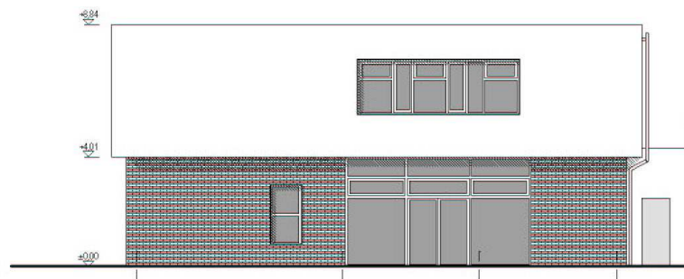
Ansicht Osten
