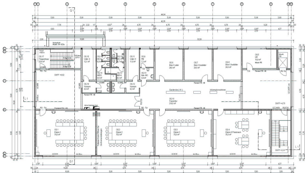
Obergeschoss
