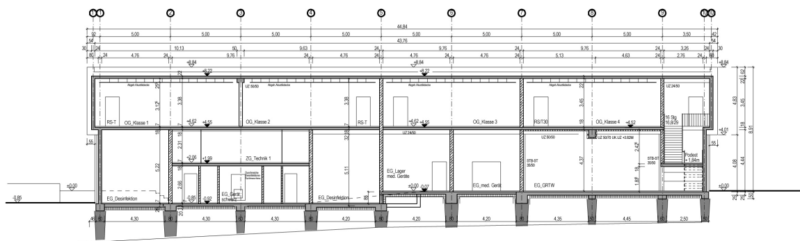
Längsschnitt L1 - L1
