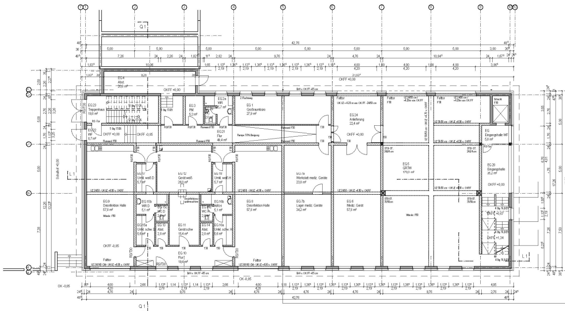
Erdgeschoss
