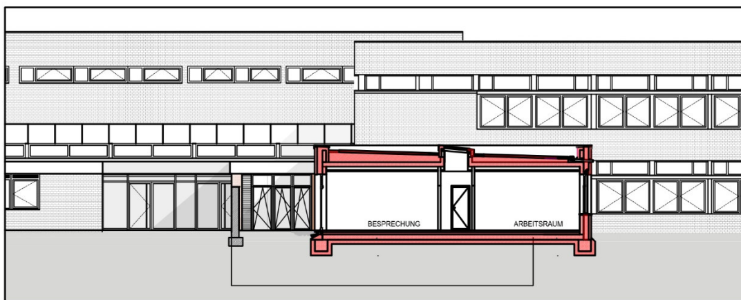
Schnitt B-B
