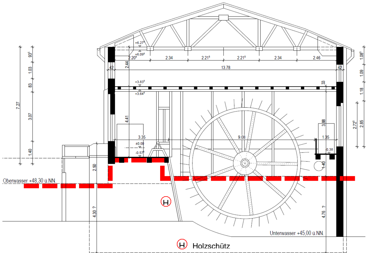
Schnitt Wasserrad
