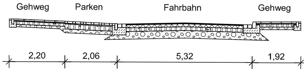
Schnitt A - A
