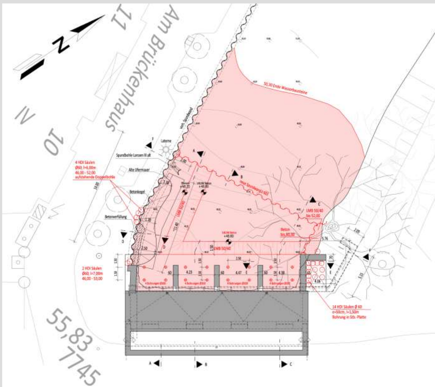
Brückenhaus „Leineinsel Döhren“ - Grundriss -
