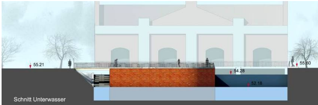
Abb. 5: Schnitt durch das Unterwasser zwischen der geplanten Wasserkraftanlage und der Brückstraße, Blick nach Süden
