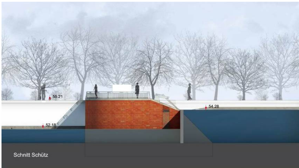
Abb. 7: Schnitt durch das Wehr westlich der geplanten Wasserkraftanlage
