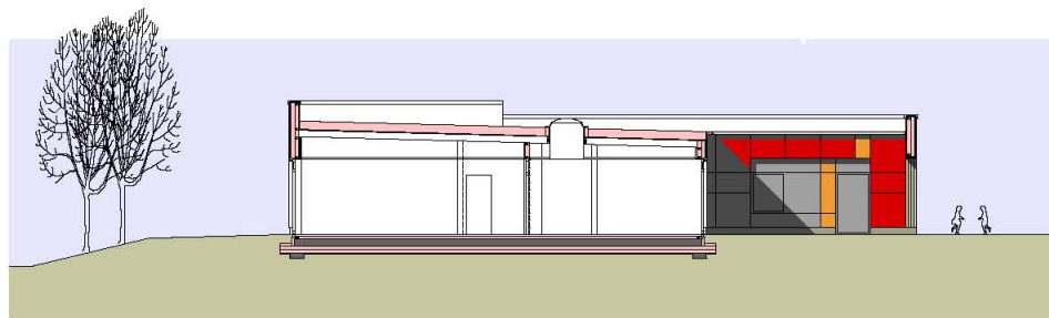
SCHNITTANSICHT 1-1
