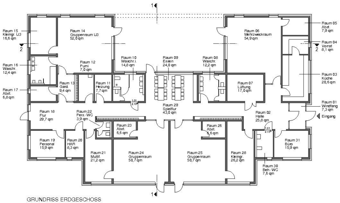
GRUNDRISS ERDGESCHOSS
