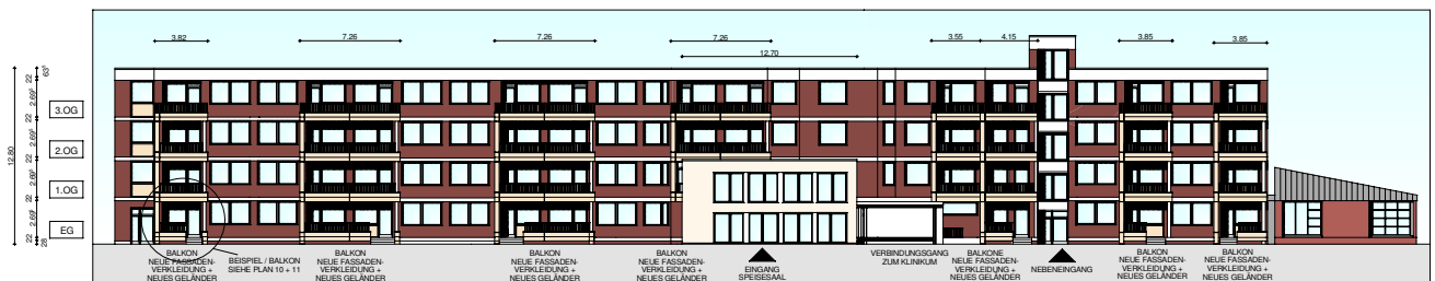
ANSICHT WESTEN
