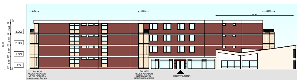
ANSICHT NORDEN
