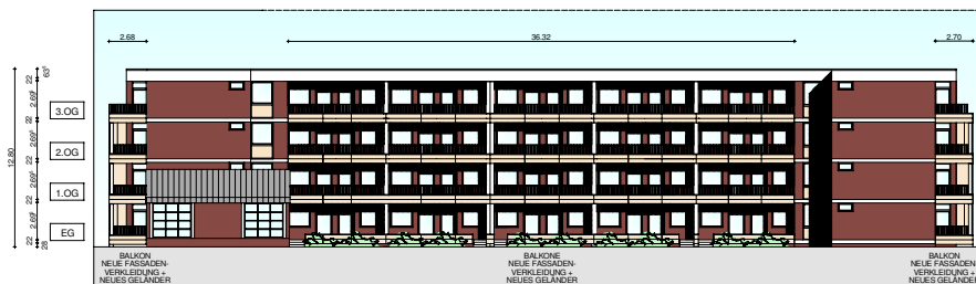
ANSICHT SÜDEN
