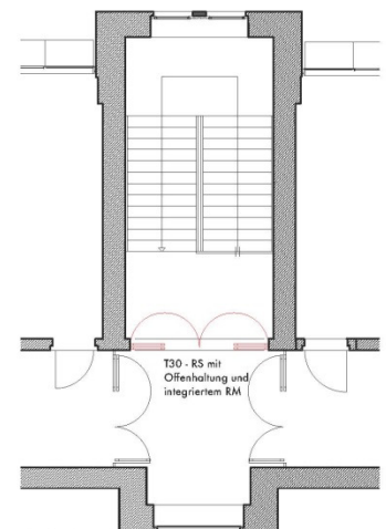
GRUNDRISS DG
