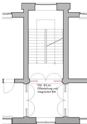
GRUNDRISS 1.OG
