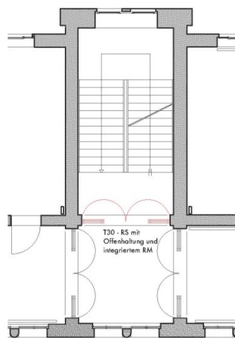
GRUNDRISS 2.OG
