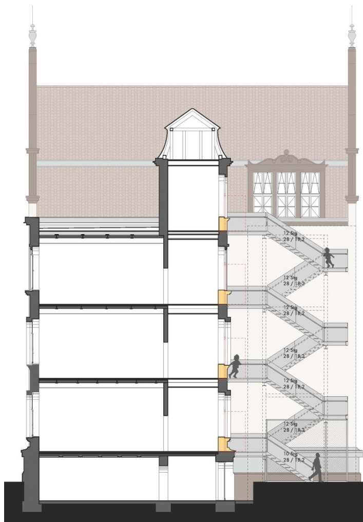
SCHNITT A-A
