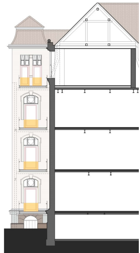
SCHNITT B-B
