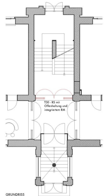
GRUNDRISS EG
