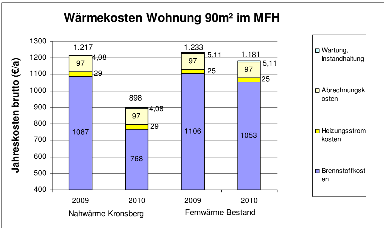
Abb. Typische Wärmekosten (incl. MWSt.) einer Wohnung (90 m 2 ) im Mehrfamilienhaus am Kronsberg und im hannoverschen Durchschnitt (Durchschnitt nach Heizspiegel Hannover) in den Jahren 2009 und 2010
