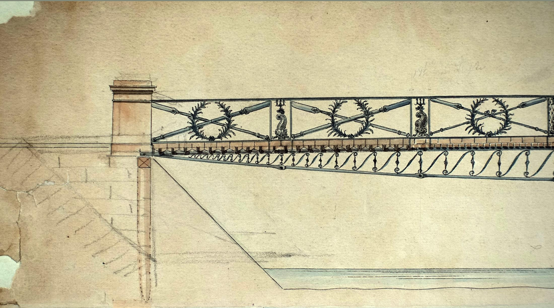
Laves Brücke Ansicht
