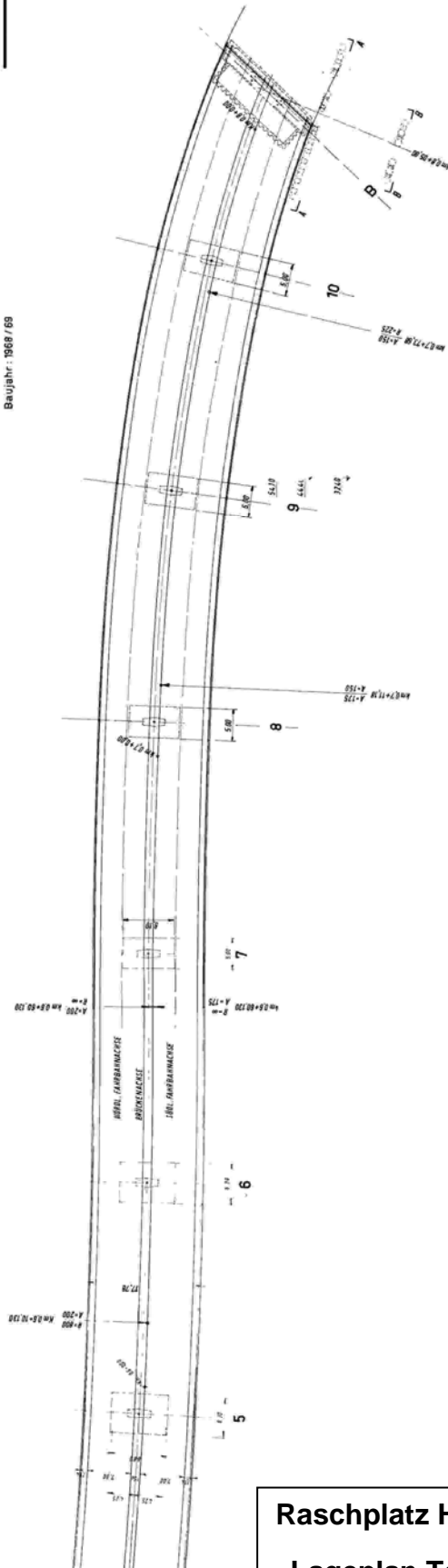
FAHRBAHN - DRAUFSICHT
