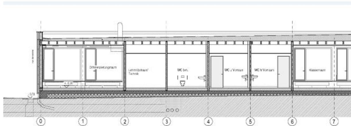
Schnitt B-B
