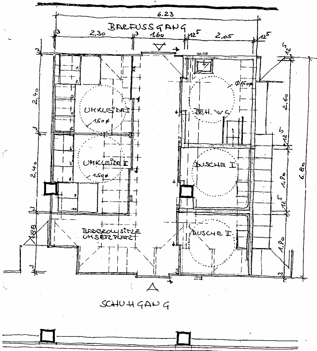
GRUNDRISS 1:50
