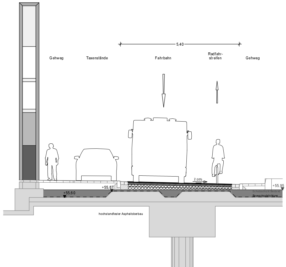
Schnitt 2 Fahrbahnerneuerung (mit aufgehellter Oberfläche mit Natursplitt auf Epoxidharz)
