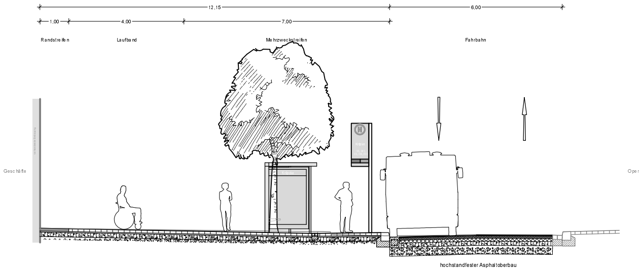
Schnitt 1-1 Bushaltestelle und Fahrbahn in Asphalt
