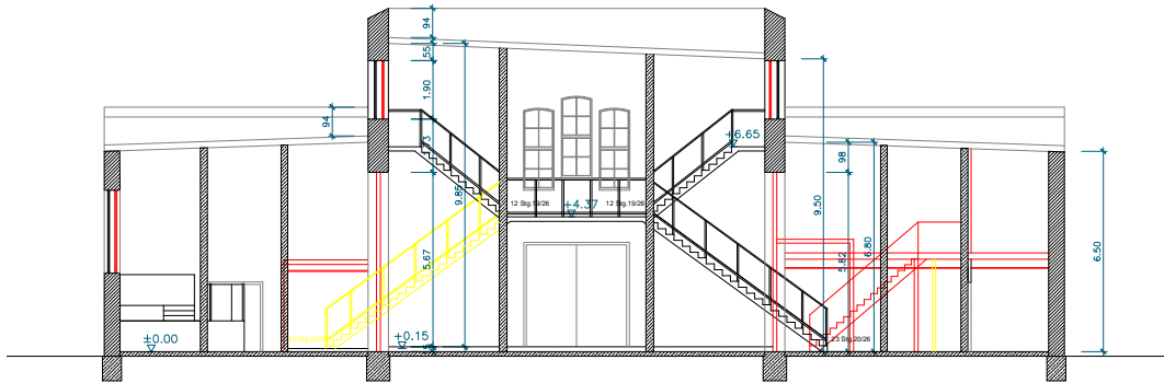
Schnitt B-B
