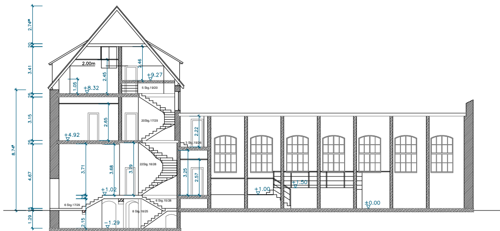
Schnitt A-A
