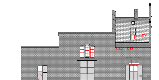
ANSICHT OST
