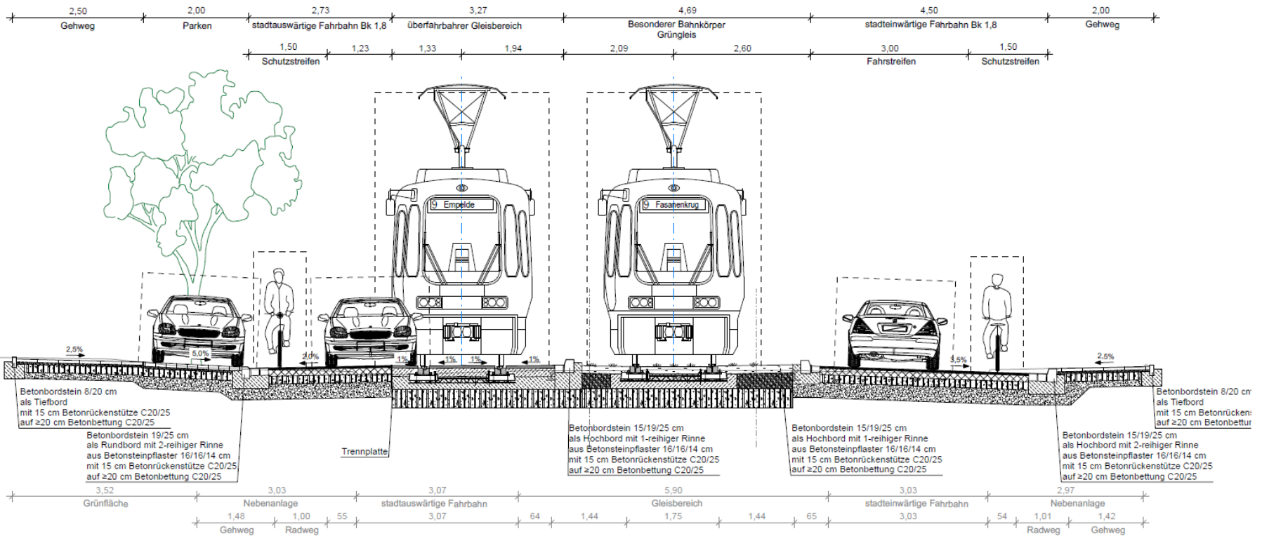
Ausbauquerschnitt 2 (200+775,766)
