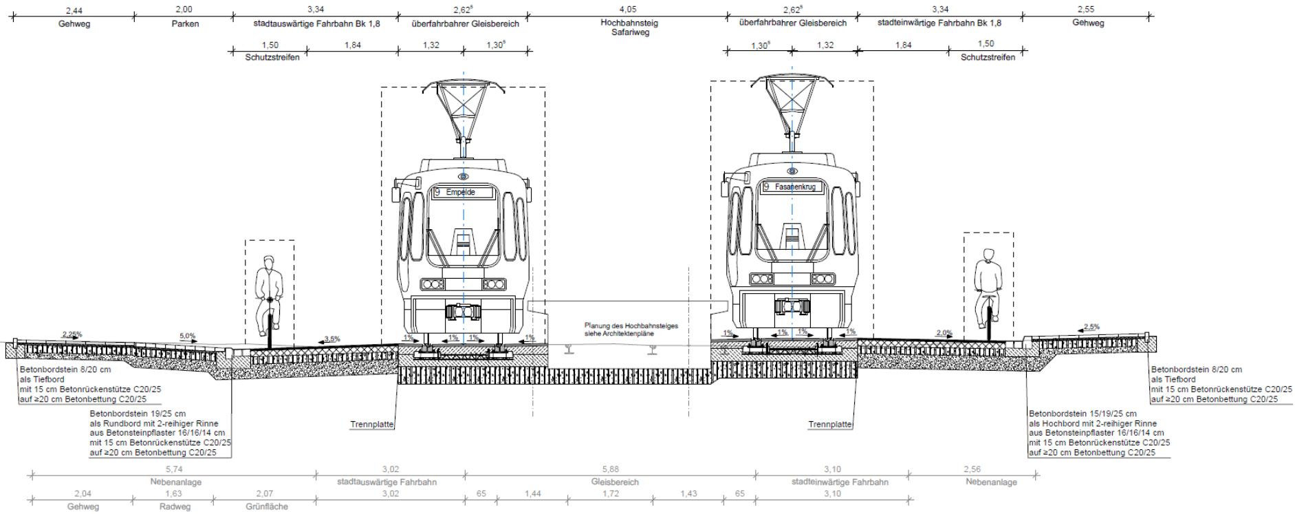
Ausbauquerschnitt 3 Hochbahnsteig (200+574,641)
