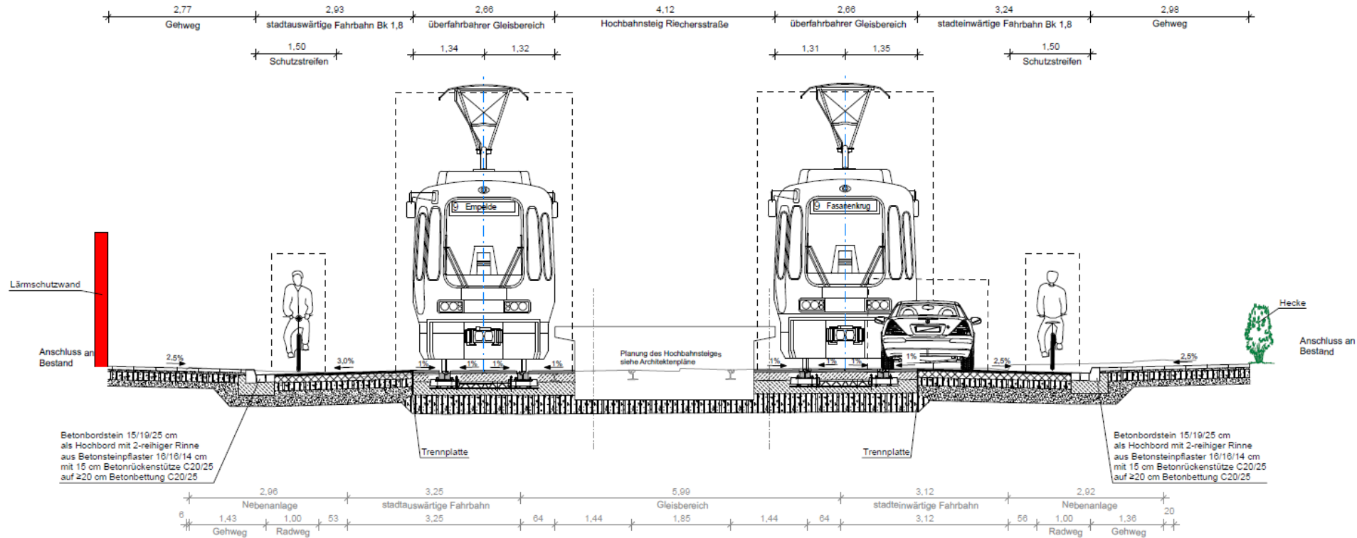
Ausbauquerschnitt 1 Hochbahnsteig (200+930,302)
