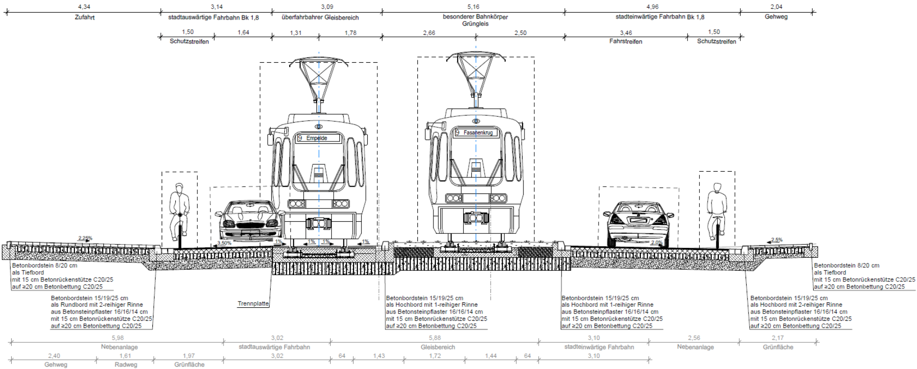
Ausbauquerschnitt 4 (200+461,600)
