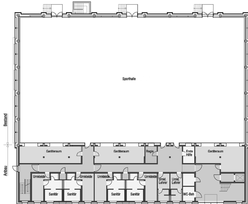
Anbau Sporthalle / NTW Grundriss EG
