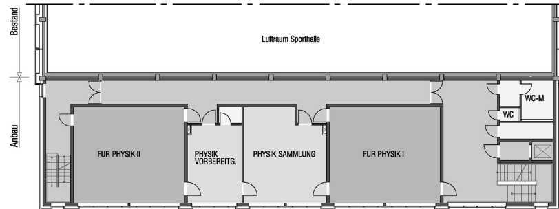
Anbau Sporthalle / NTW Grundriss 1. OG
