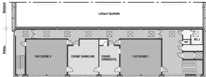
Anbau Sporthalle / NTW Grundriss 2. OG
