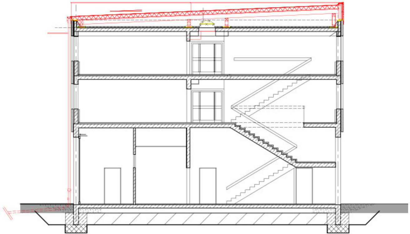
Schnitt Fahrzeughalle/Wachgebäude
