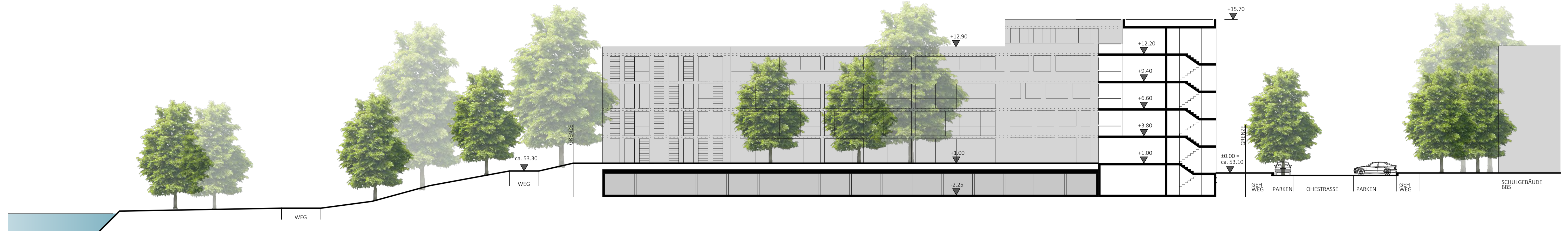
SYSTEMSCHNITT OHESTRASSE M 1:200
