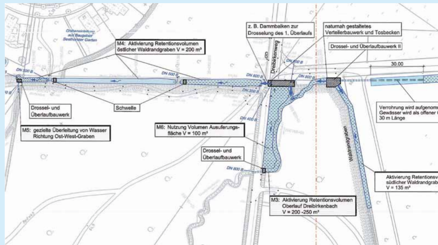
Abb. 17 : Ausschnitt aus dem Lageplan „Retentionsmaßnahmen Seelhorstwald“ (Plan: Stadtentwässerung Hannover)
