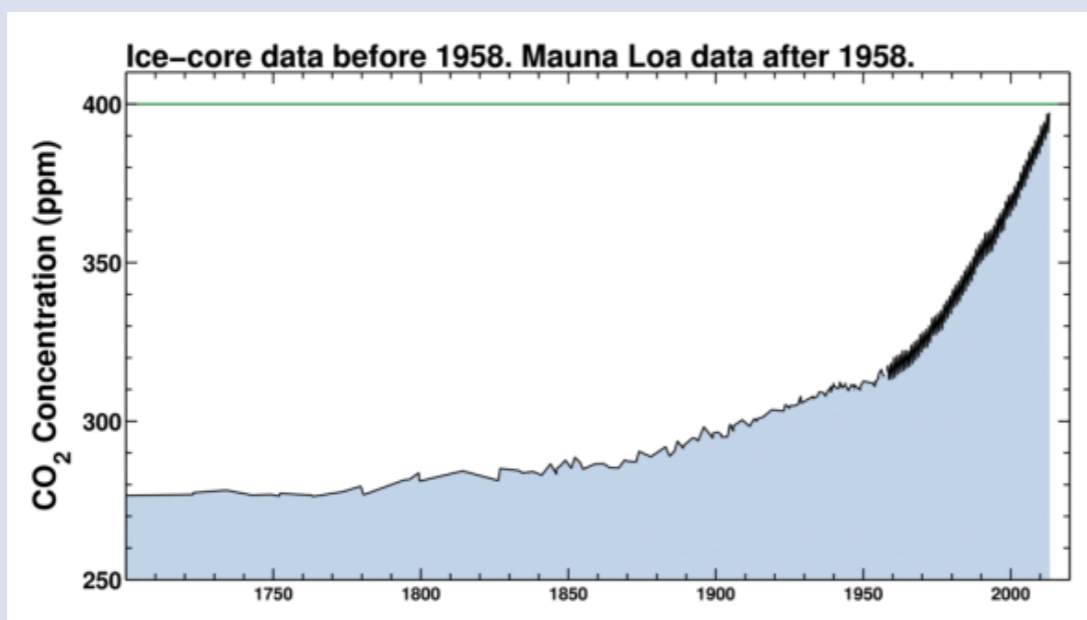
Abb. 2: Die atmosphärische CO 2 -Konzentration seit dem Jahr 1700. Daten der NOAA (National Oceanic and Atmospheric Administration) aus Hawaii seit 1958, davor Berechnung anhand von Eisbohrungen. (Copyright/Quelle: Scripps Institution of Oceanography, UC San Diego)
