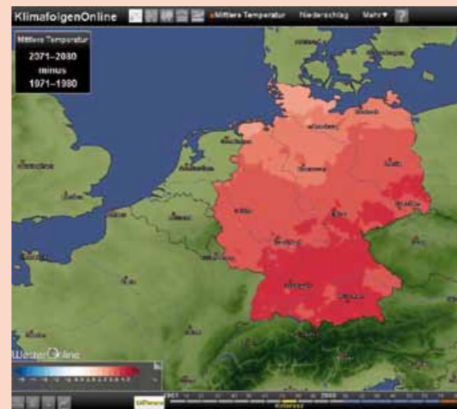
Abb. 3: Ein Vergleich der Jahresdurchschnittstemperaturen der 1970er Jahre mit denen, die für die 2070er Jahre in Deutschland erwartet werden, zeigt einen deutlichen Anstieg – im Durchschnitt eine Zunahme von 3,5 °C innerhalb von 100 Jahren. (Quelle: KlimafolgenOnline.de)
