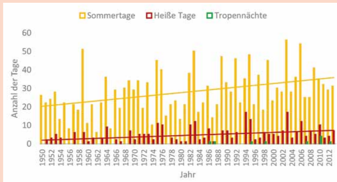
Abb. 4: Anzahl von Sommertagen (gelb), Hitzetagen (rot) und Tropennächten (grün) in Hannover-Langenhagen in den Jahren 1950 bis 2013 (Quelle: Meteoterra/GEO-NET, 2015)
