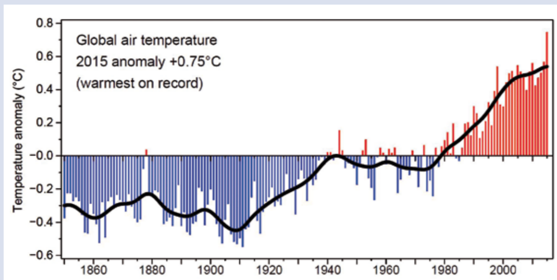
Abb. 1: Abweichungen des globalen Mittels der bodennahen Lufttemperatur vom Mittelwert im Referenzzeitraum 1961 – 1990 (rote und blaue Balken), die durchgezogene schwarze Linie stellt den nichtlinearen Trend dar (Quelle: Climate Research Unit, University of East Anglia, 2015)
