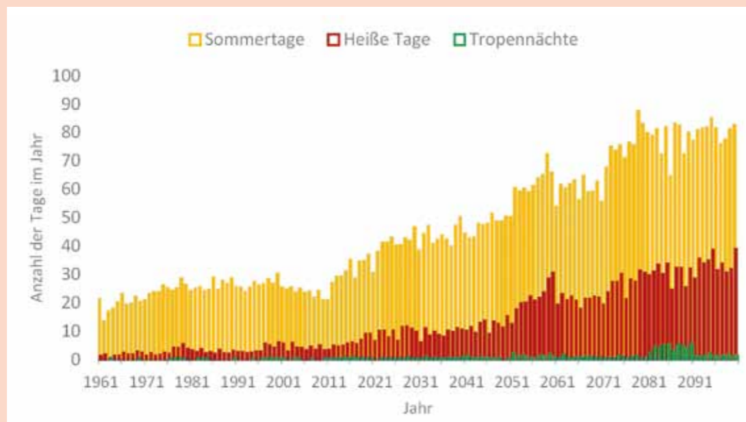
Abb. 5: Modellerte Anzahl von Sommertagen (gelb), Hitzetagen (rot) und Tropennächten (grün) für Hannover-Langenhagen im Zeitraum 1961 – 2100 (Datenbasis: WETTREG 2010, Szenario A1B, Mittel über zehn Modellläufe) (Quelle: Meteoterra/GEO-NET, 2015)
