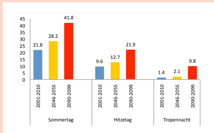
Abb. 8: Mittlere jährliche Häufigkeit klimatologischer Ereignisse in der Innenstadt von Hannover für die Zeithorizonte 2001 bis 2010, 2046 bis 2055 und 2090 bis 2099 (Datenquelle: GEO-NET 2011)
