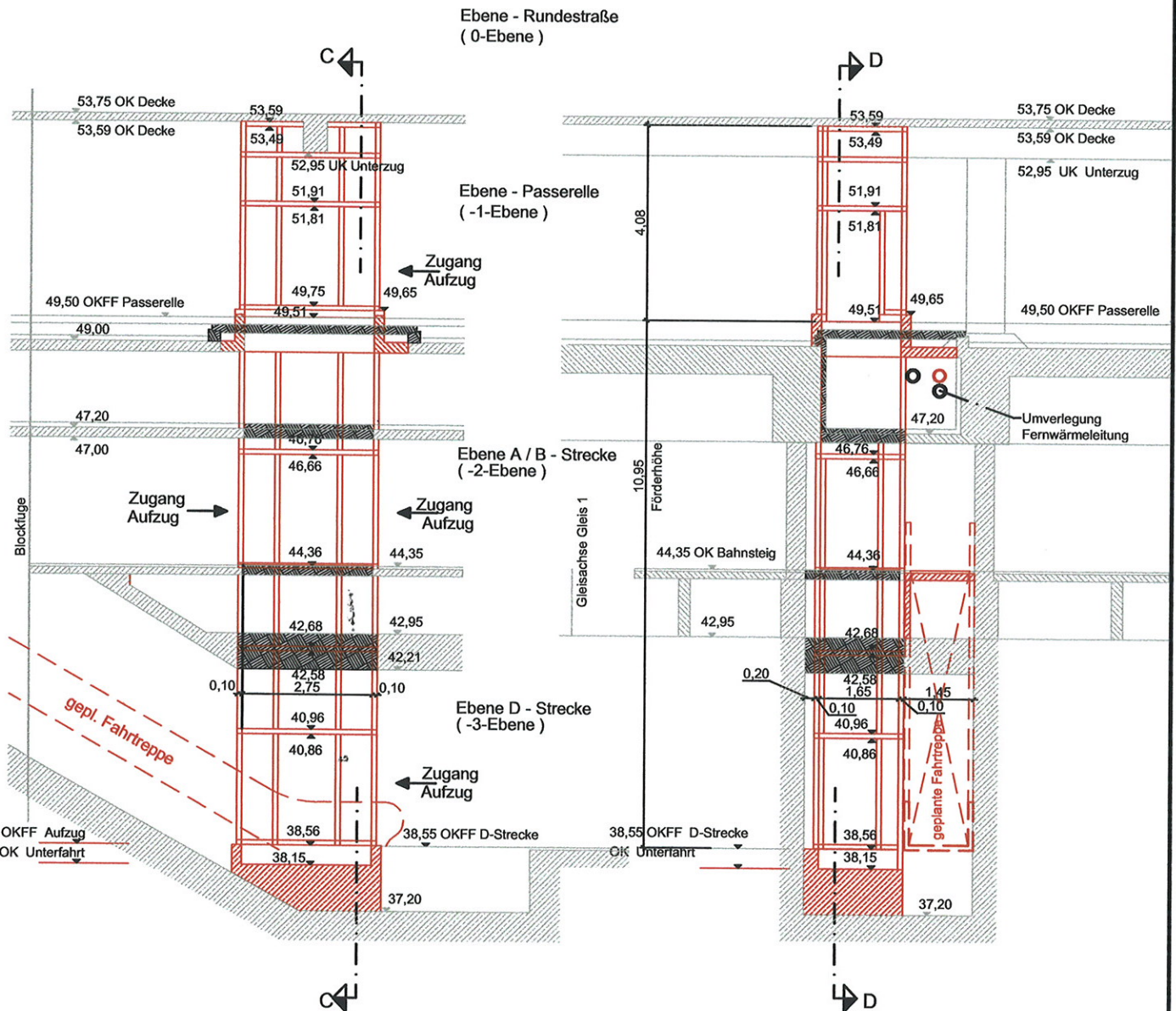
Schnitt C - C
